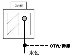
ブレーキカプラー配線 常時電源
