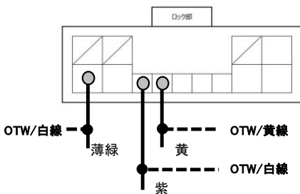
アンロック信号への接続
